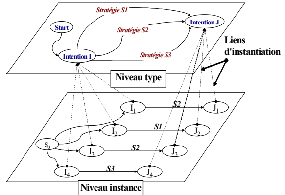
Figure 4. Les niveaux d'abstraction du map
