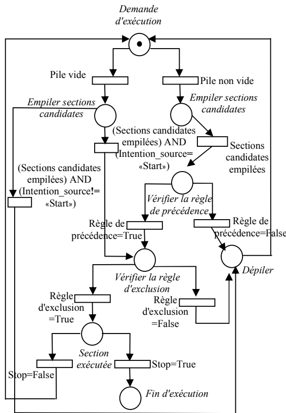
Figure 8. Fonctionnement de la pile de sections
