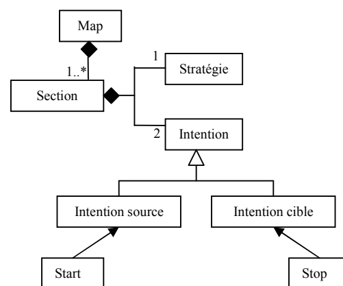
Figure 2. Méta-modèle du map
