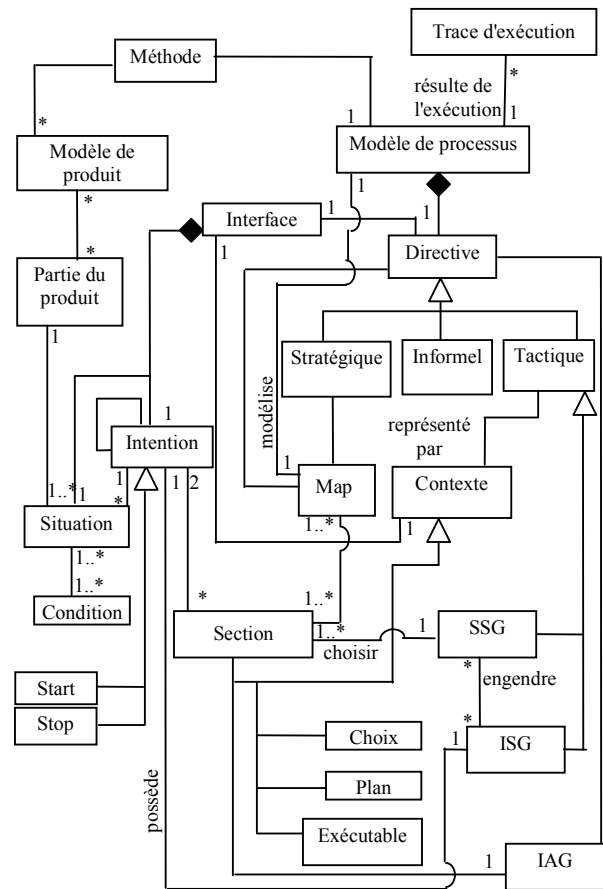
Figure 1. Le méta-modèle NATURE
