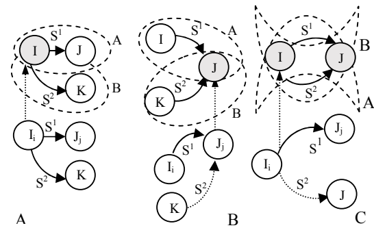
Figure 12. La règle d'exclusion
