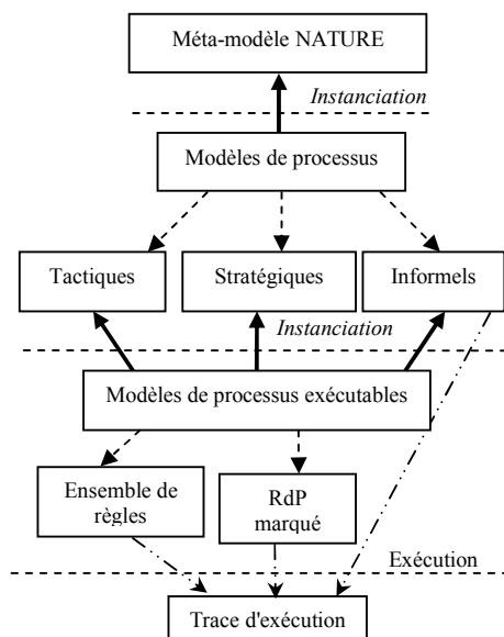
Figure 6. Evolution d'un modèle de processus dans un ECP
