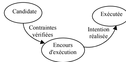
Figure 9. Les états d'une section du map
