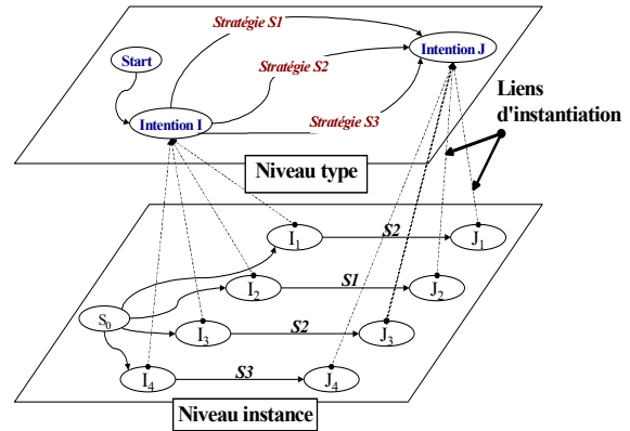
Figure 4. Les niveaux d'abstraction du map
