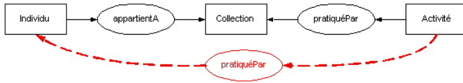
FIG. 6 – Une règle d'inférence : la connaissance ajoutée est en pointillés.
