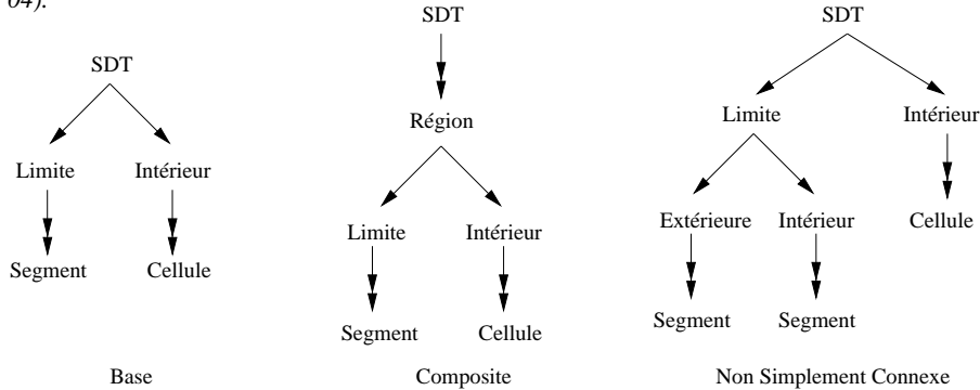
Figure 1. Graphe des constructeurs pour les représentations spatiales
