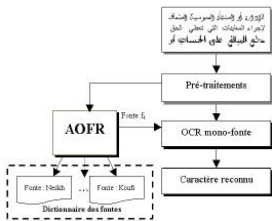
FIG. 3. Schéma global d'un système AOCR multifonte doté d'un module OFR en amont.
