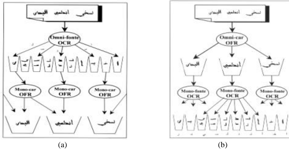
FIG 1- stratégies de combinaison de l’OFR avec l’OCR, (a) a posteriori, (b) a priori, [Gazzah 03a].
