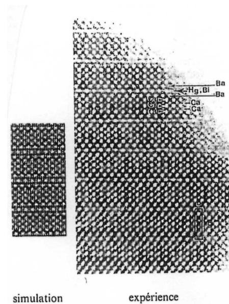
Fig. 3. Image MET de la structure d'un composé au mercure 1223 supraconducteur à environ 120 ° K. Comparaison avec l'image simulée numériquement à partir d'un modèle de structure cristalline (Doc. : M.-Y. Hervieu – Caen).
